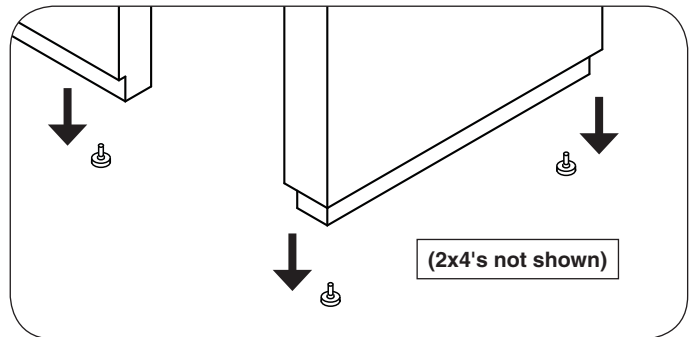
Fig. 2-2 Remove Levelers
