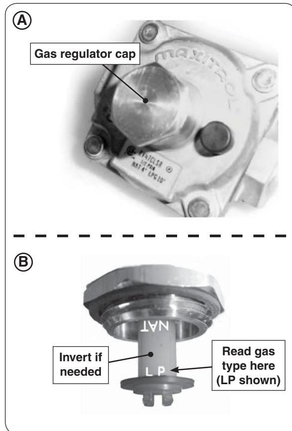
Fig. 25-1 Convert regulator
