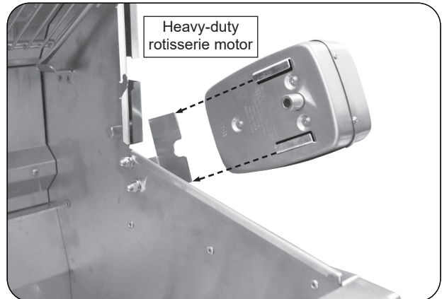
Fig. 39-2 Install rotisserie motor
