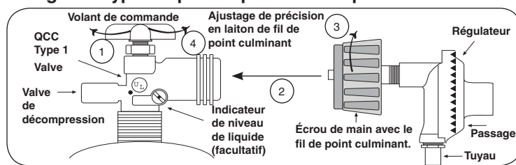
Fig. 18-1 type coupleur rapide de fil de point culminant d'I
