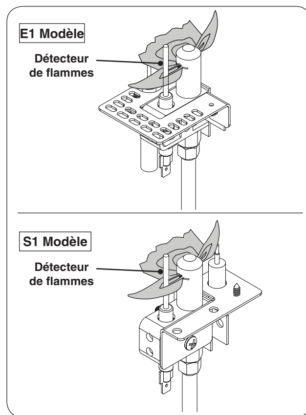
Fig. 32-2 Bonne flamme pilote
